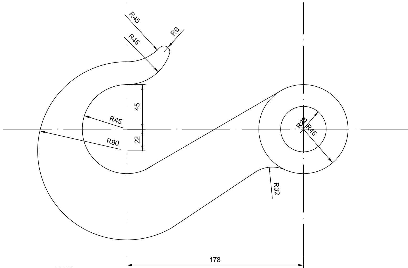
HOOK Scale: 1:2
